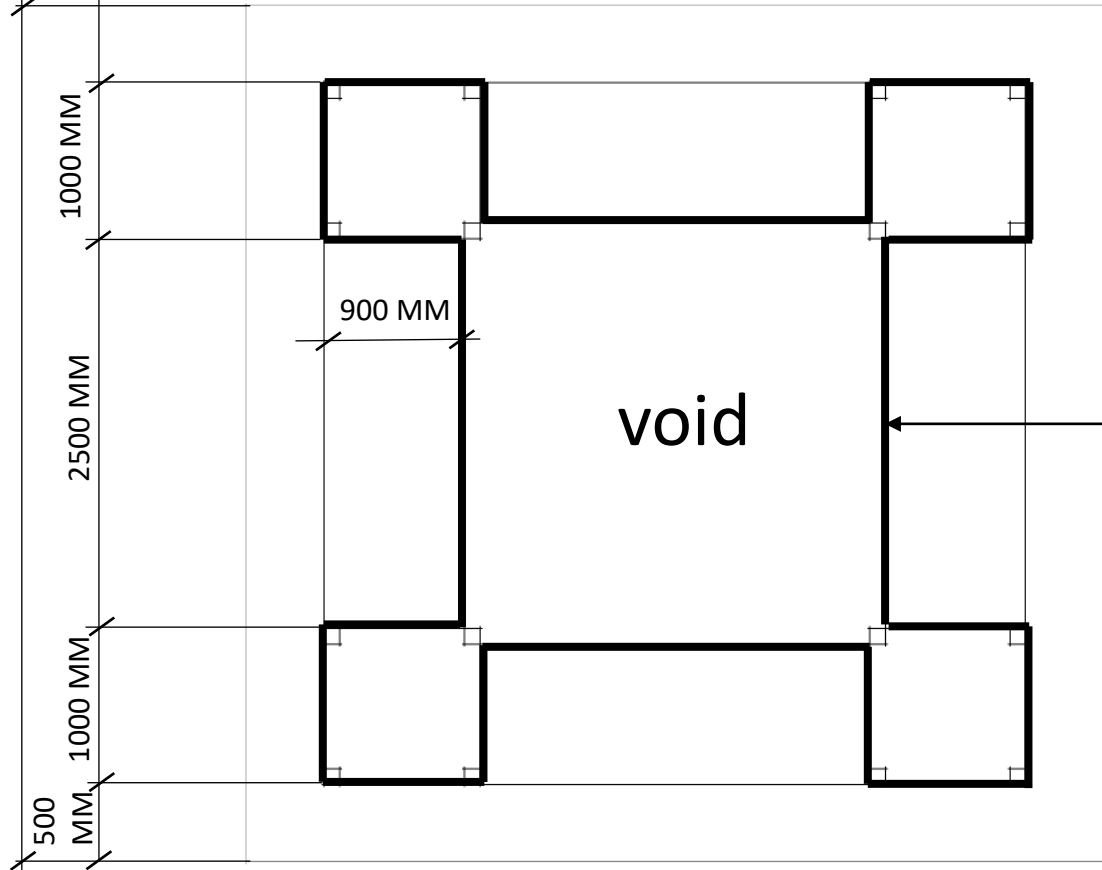
D 1 PLAN SCALE: N.T.S
