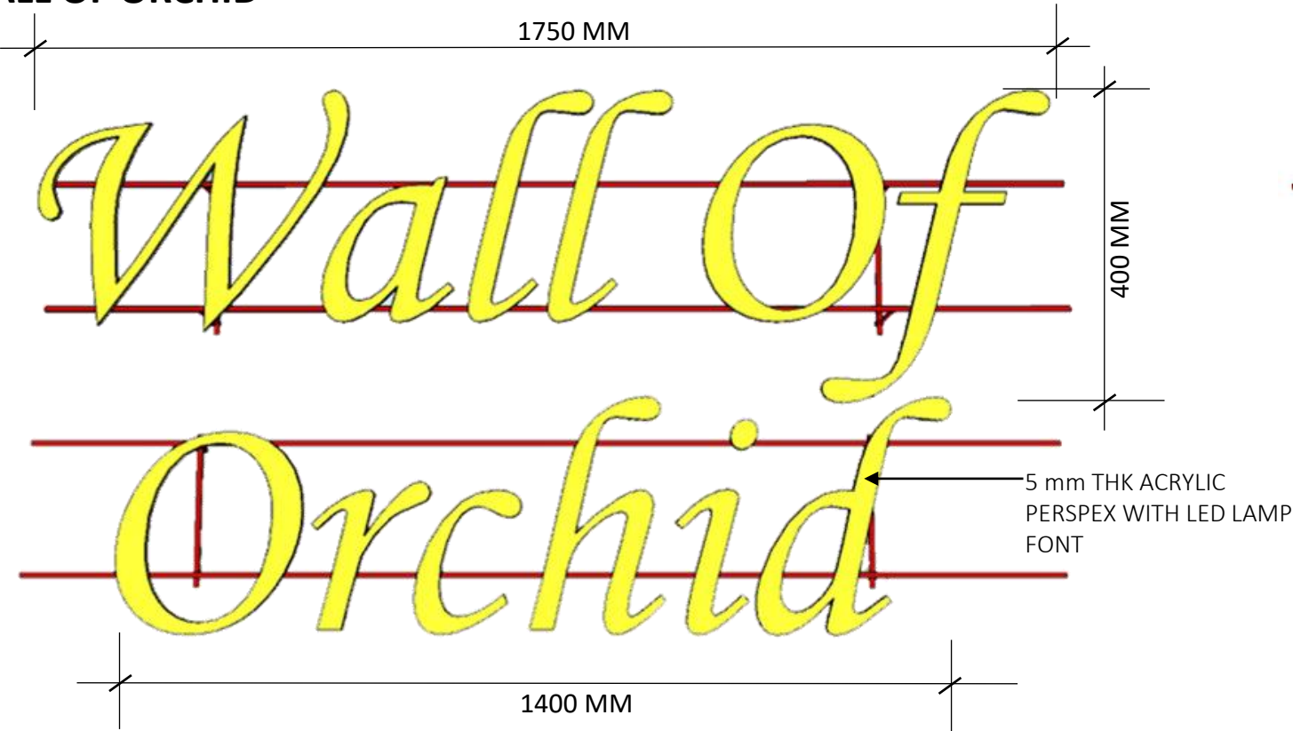
E 1 FRONT VIEW SCALE: N.T.S
