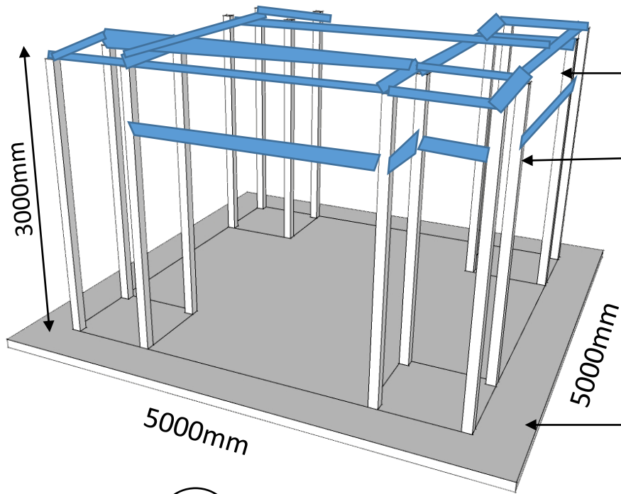
D 3 PERSPECTIVE SCALE: N.T.S
